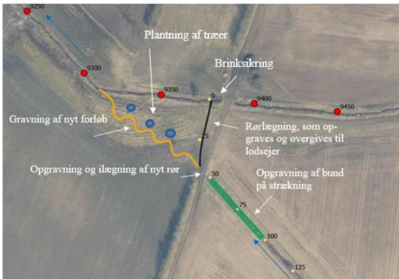
Figur 1. Figuren viser den gamle rørlægning (sort streg) og det nye forløb (gul streg). Placeringen af træer er vist med blå cirkler.
