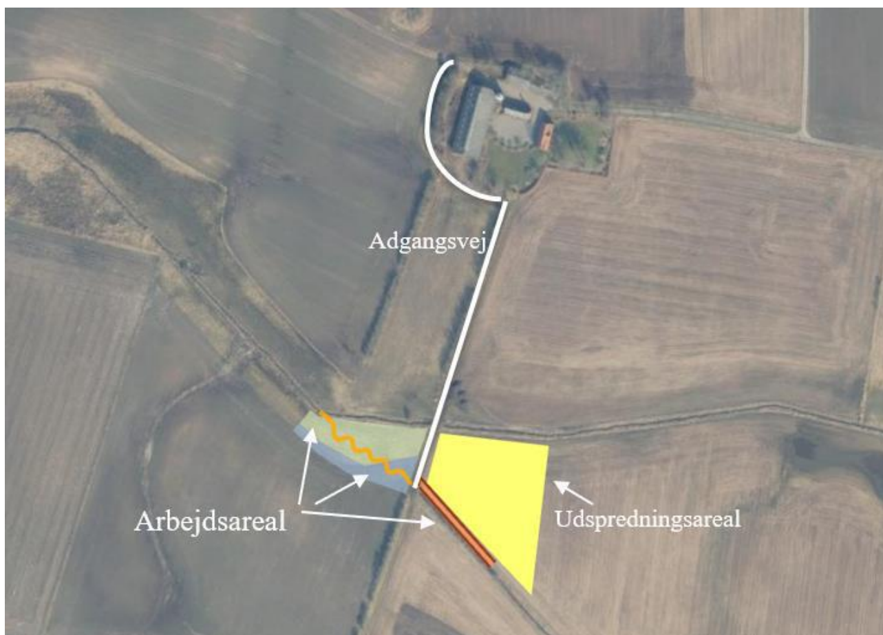
Figur 2. Oversigt over arbejdsarealer og udspretningsarealer for overskudsjord. Arealerne er estimeret og kan variere en smule i størrelse.
